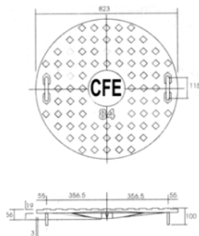
Marco y Tapa CFE P84 A con Bisagra fierro fundido de 185 kg.
