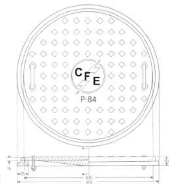
Aro y tapa CFE 84A fierro fundido de 255 kg.
