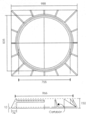
Marco y tapa CFE P84 A fierro fundido de 255 kg.
